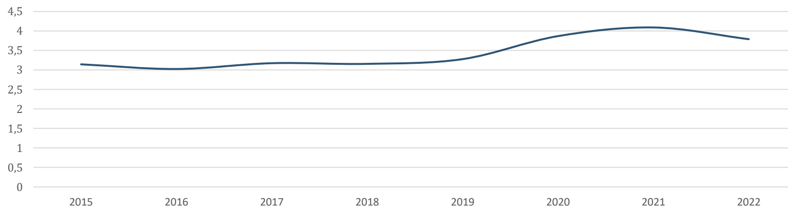
Indice linéaire de volume non compté (m³/km/jour)
